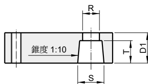
單邊壓板安裝尺寸
