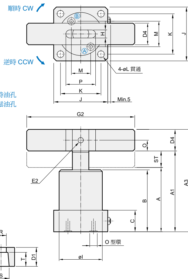
單邊壓板安裝尺寸
