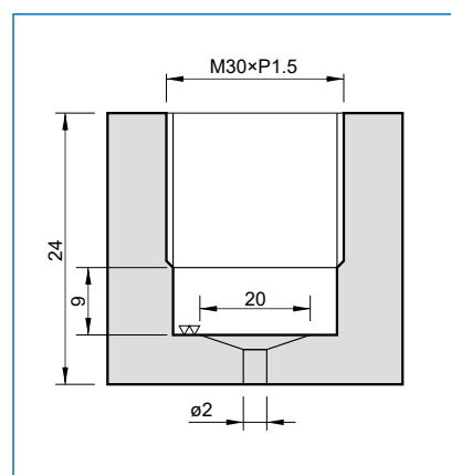
建議安裝尺寸
