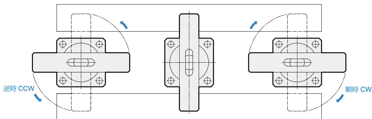
壓板鎖緊操作方式
