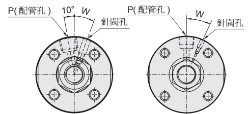
A-A 剖面
