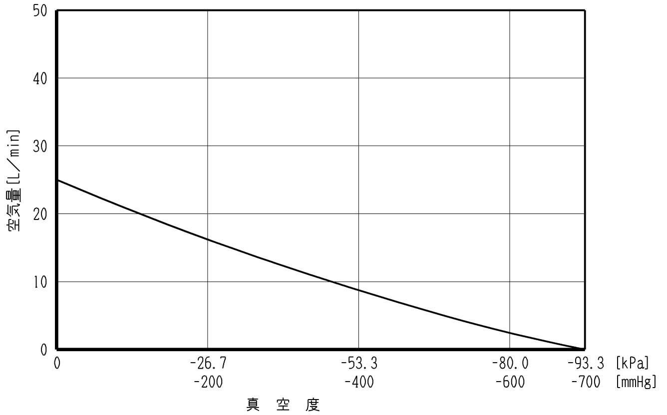
● 空気量特性図
